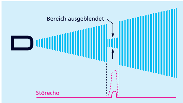
Bild 14: Prinzip der Störechoausblendung
