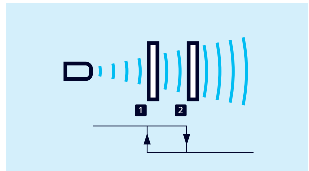
Bild 10: Hysteresebetrieb, Zweipunkt
