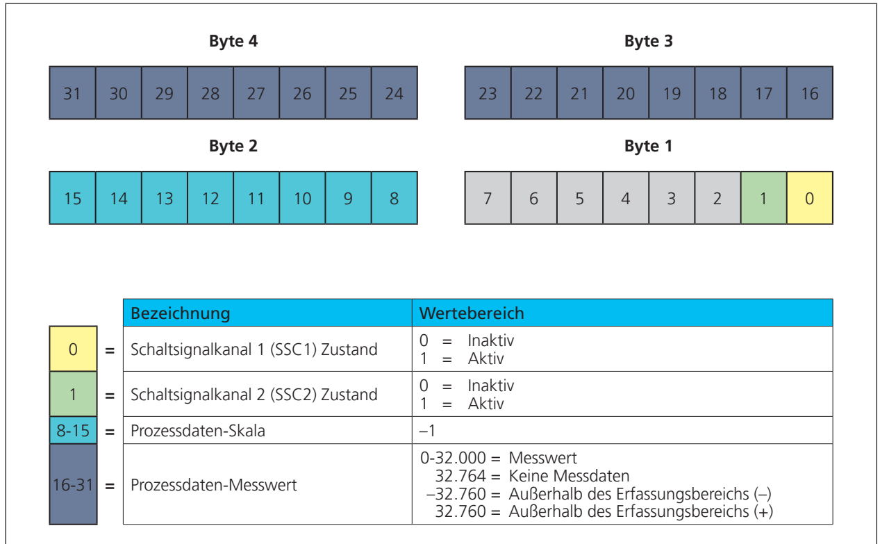
Bild 4: Aufbau der Prozessdatenstruktur
