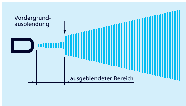
Bild 12: Messkonfiguration – Vordergrundaussblendung
