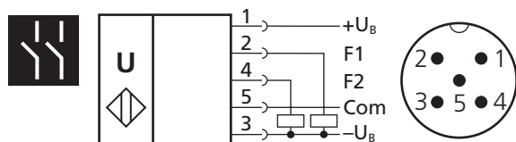
Bild 3: Anschlussbild des ucs-Sensors
