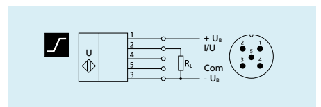
Analogausgang
