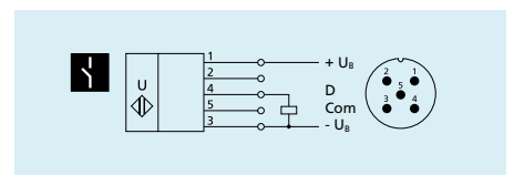
1 pnp-Schaltausgang
