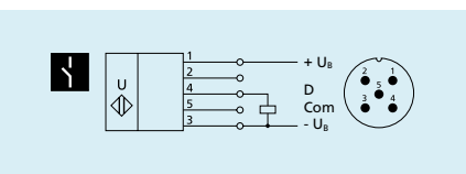
1 pnp-Schaltausgang
