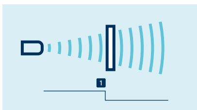
Teach-in eines Schaltpunktes
