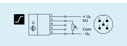
Analogausgang
