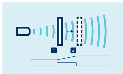
Teach-in einer Analogkennlinie bzw. eines Fensters mit zwei Schalterpunkten
