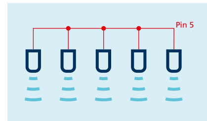
Synchronisation über Pin 5
